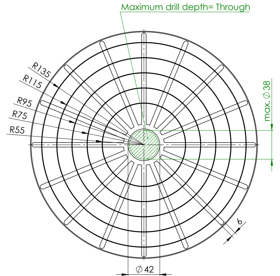
DETAIL A 2:1
