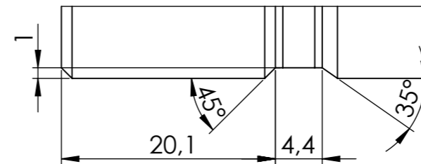
DETAIL A 2:1
